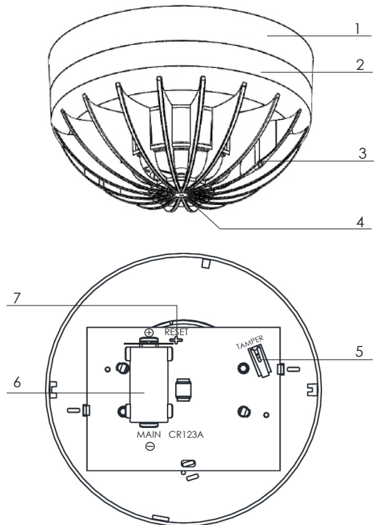
Рисунок 1 – Конструкция «Ri-SD-1»
