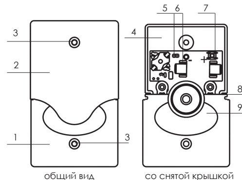
Рисунок 1 – Конструкция «Ri-S-1»
